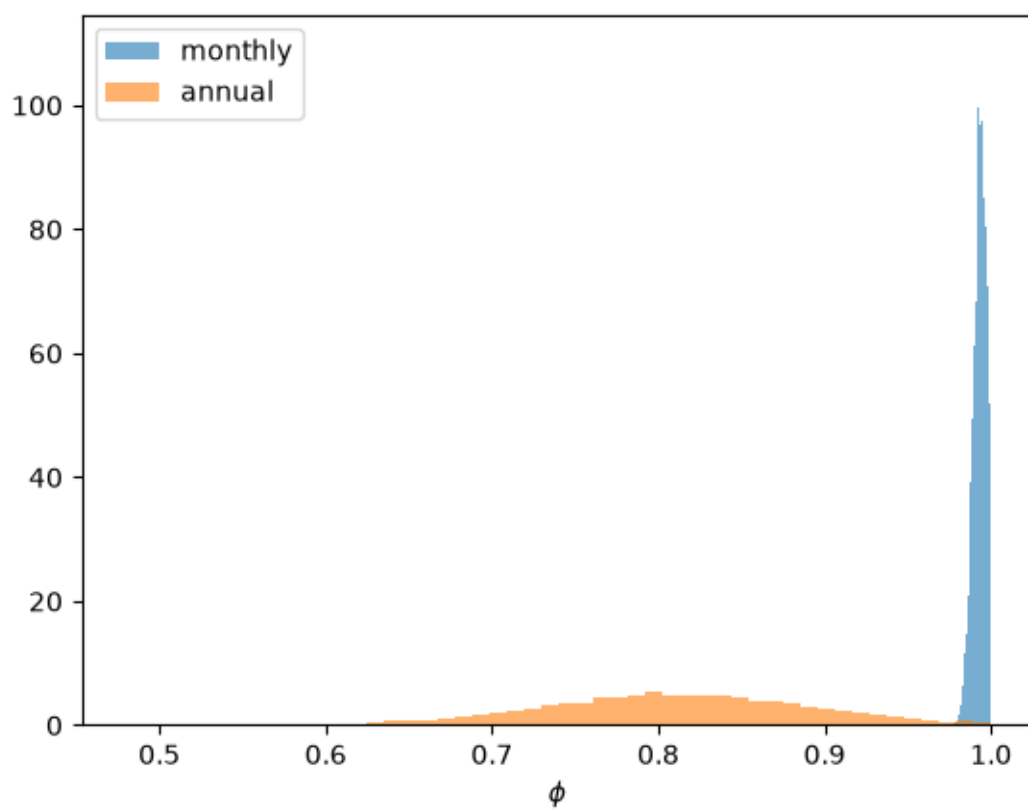
Fig. 137.3: Posterior for the persistence parameter
